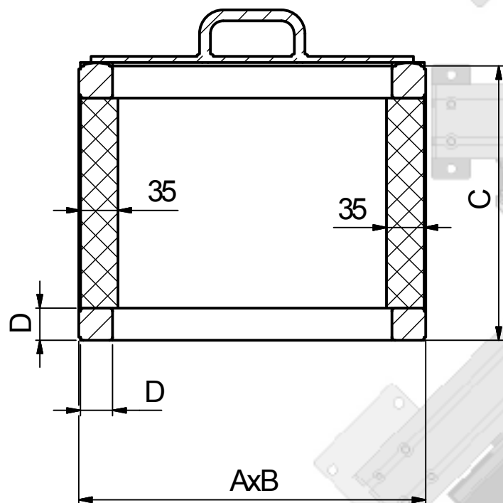
Rozměrový náčrtek
